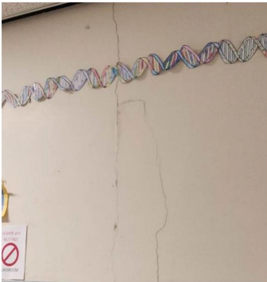
Reparaciones estructurales de paredes y suelos (Pasillos mostrados aquí)
