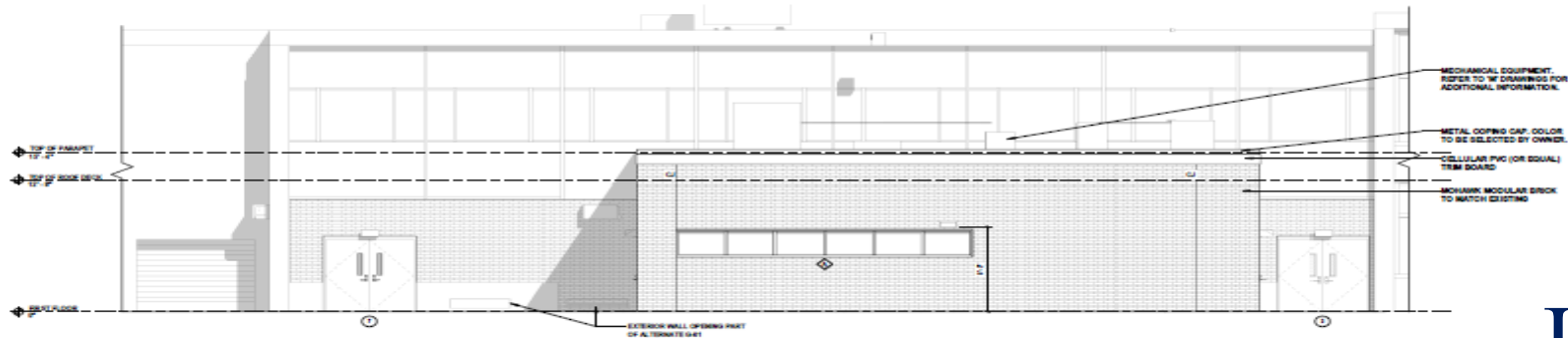
3 Exterior Elevation - East Scale: 1/8" = 1'-0"
