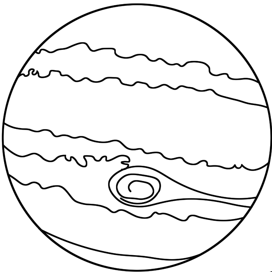
Jupiter
