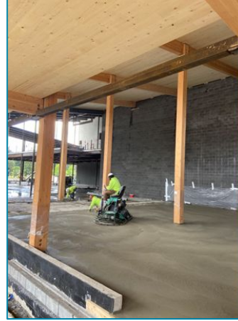
New concrete slab pour
