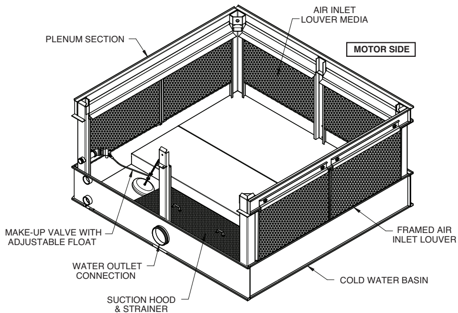
PAN & PLENUM SECTION
