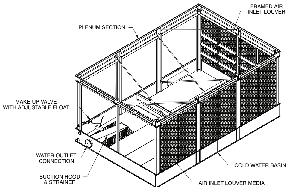
PAN & PLENUM SECTION
