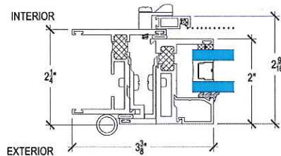
HINGED JAMB
