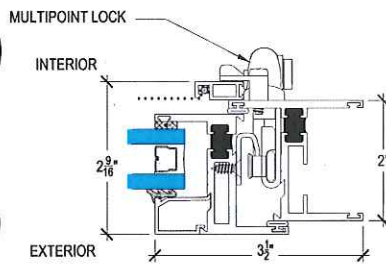
LATCH JAMB
