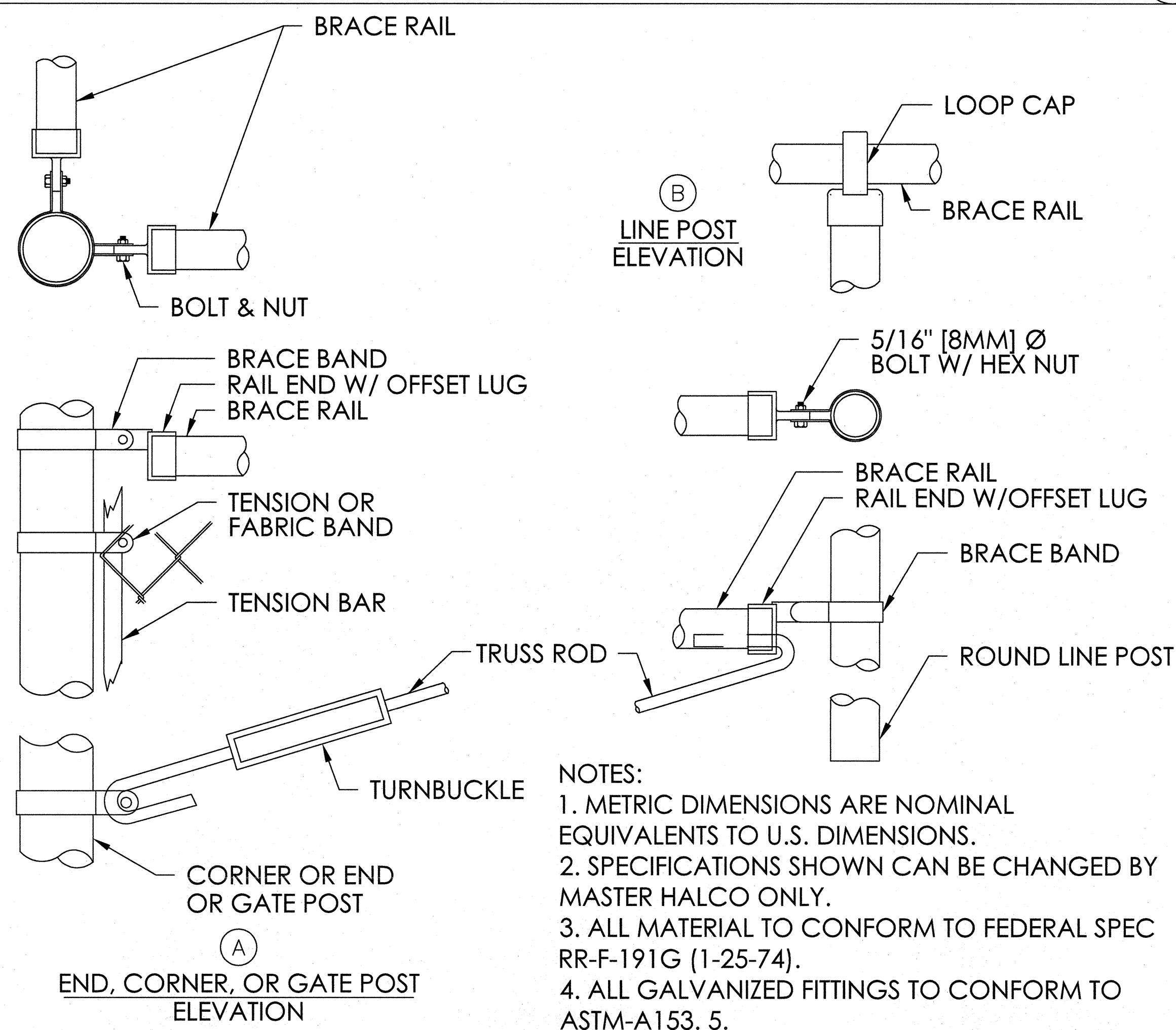
ROUND TERMINAL END POSTS 2 SCALE: 1/2"=1'-0" A-3
