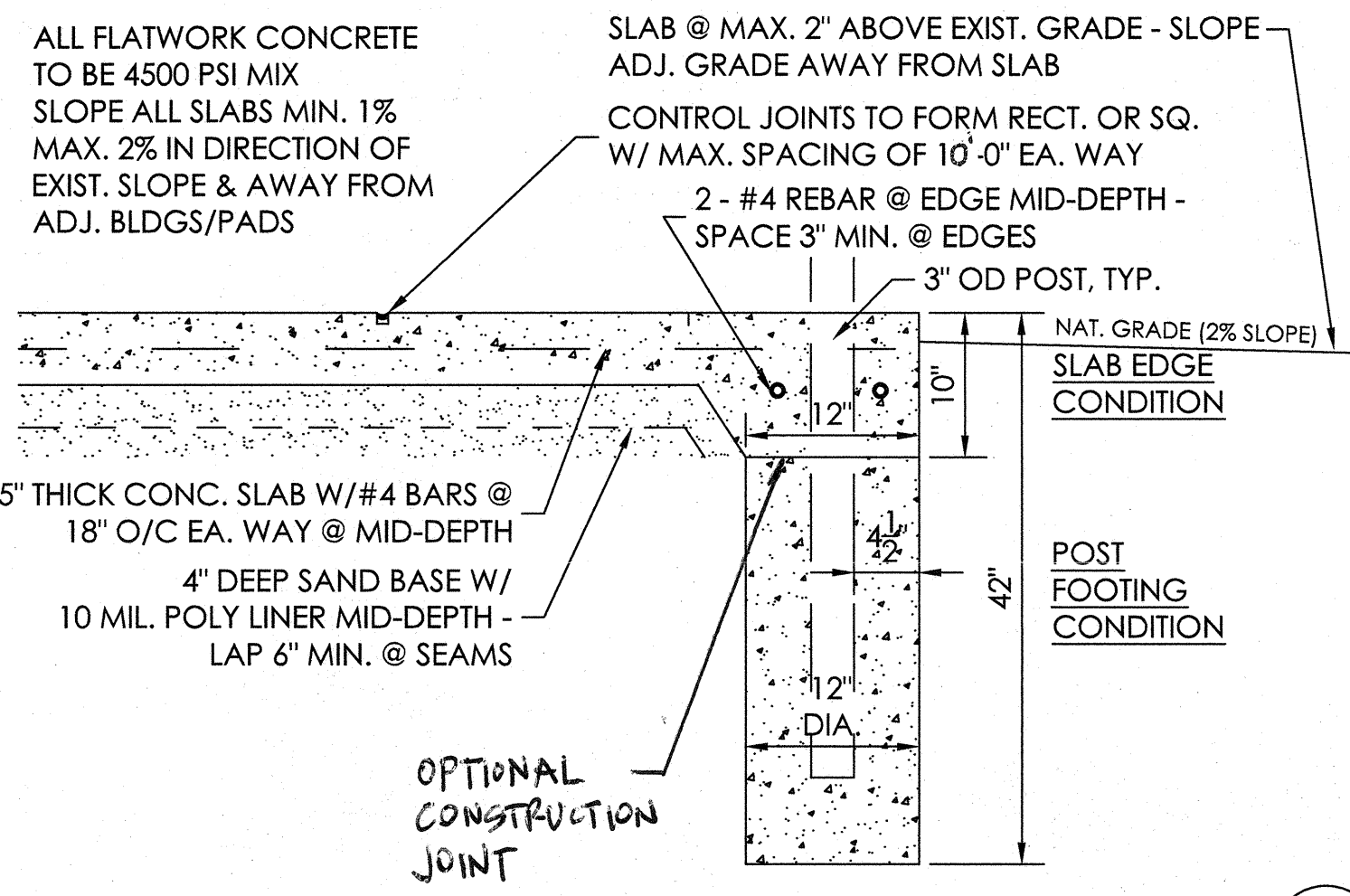
CONCRETE FLATWORK 4 SCALE: 1"=1'-0" A-3
