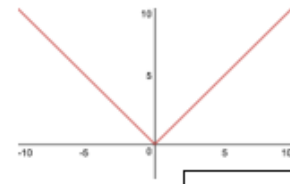
Absolute value Function f(x) = |x|
