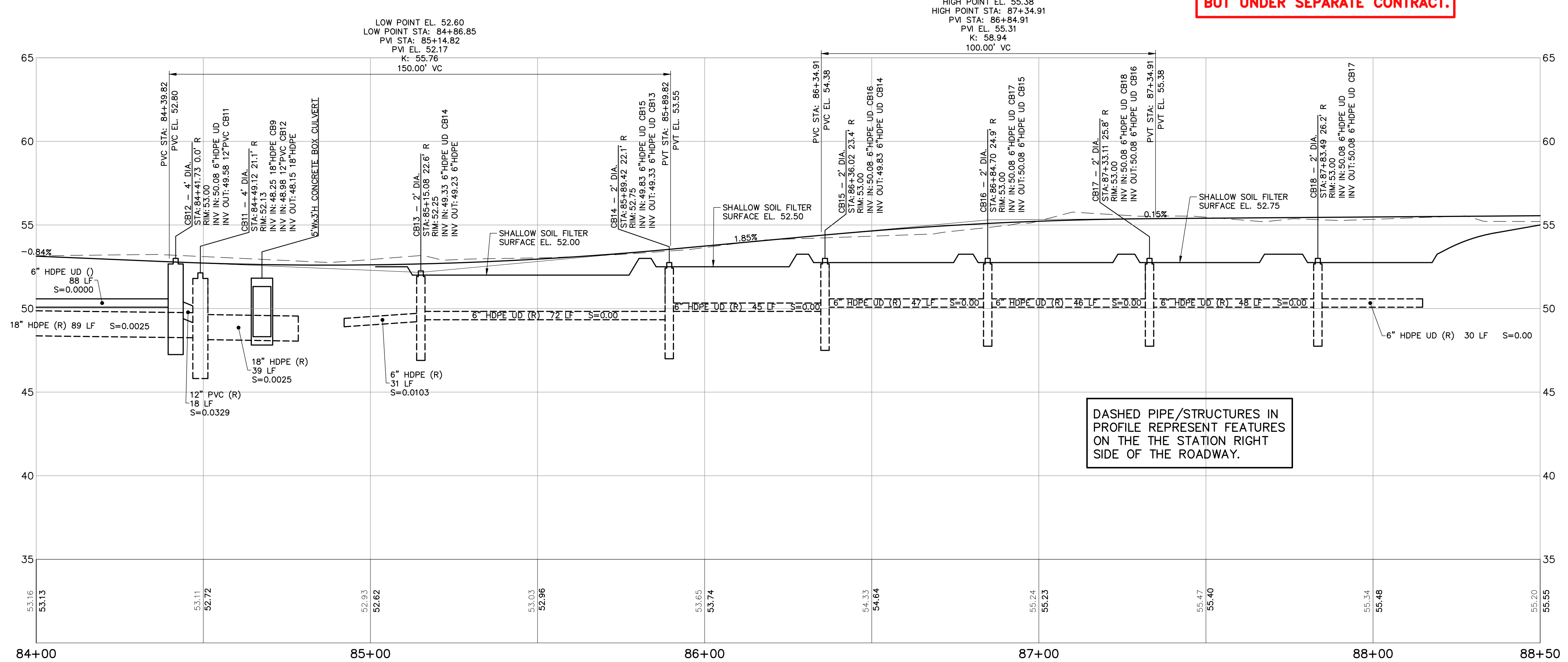
PROFILE STA. 84+00 TO STA. 88+50
