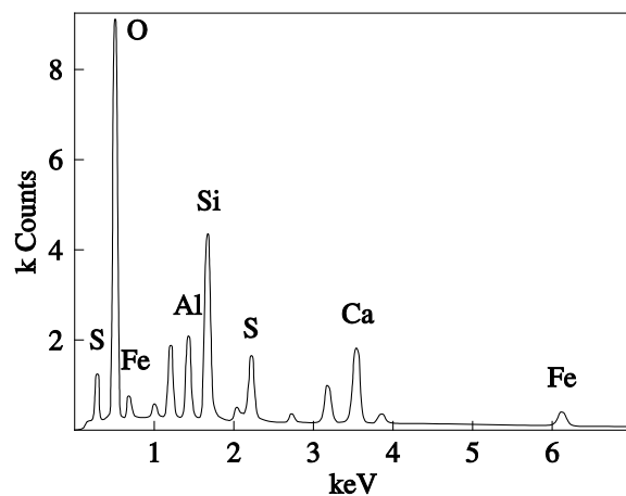
Fig. F- 3 EDS spectrum of point 2 – ettringite
