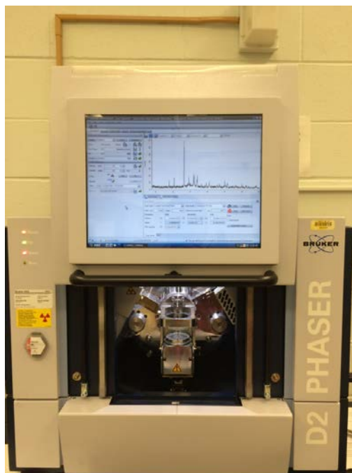
Fig. 5.2 Bruker D2 phaser X-ray diffractometer
