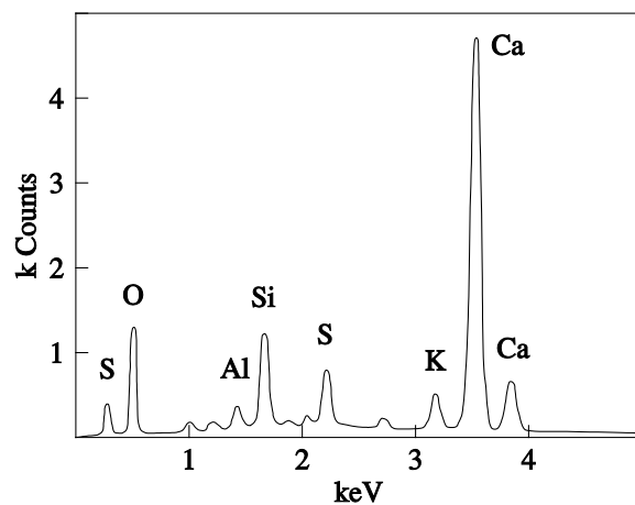
Fig. F- 6 EDS spectrum of point 5 – ettringite
