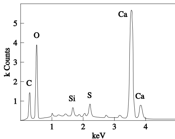
Fig. F- 5 EDS spectrum of point 4 – ettringite
