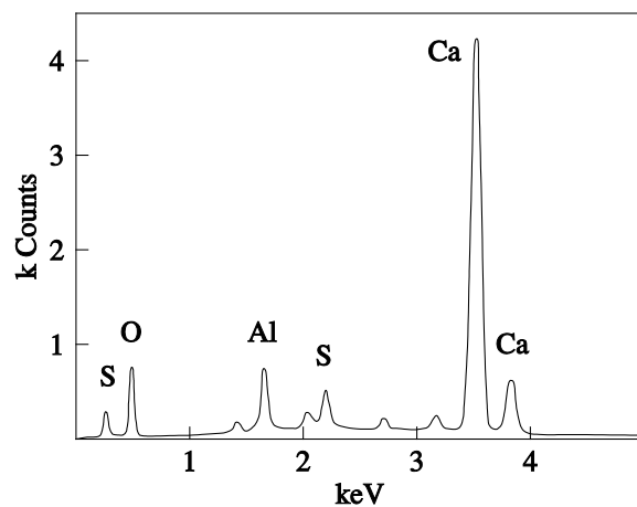
Fig. F- 7 EDS spectrum of point 6 - ettringite
