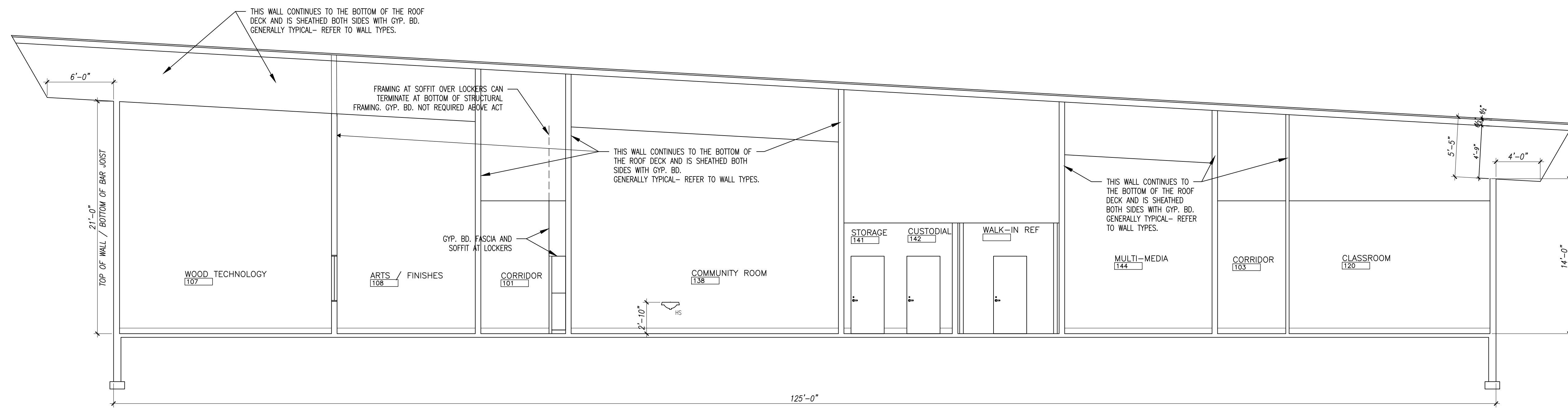
01 SECTION SCALE: 3/16" = 1'-0"
