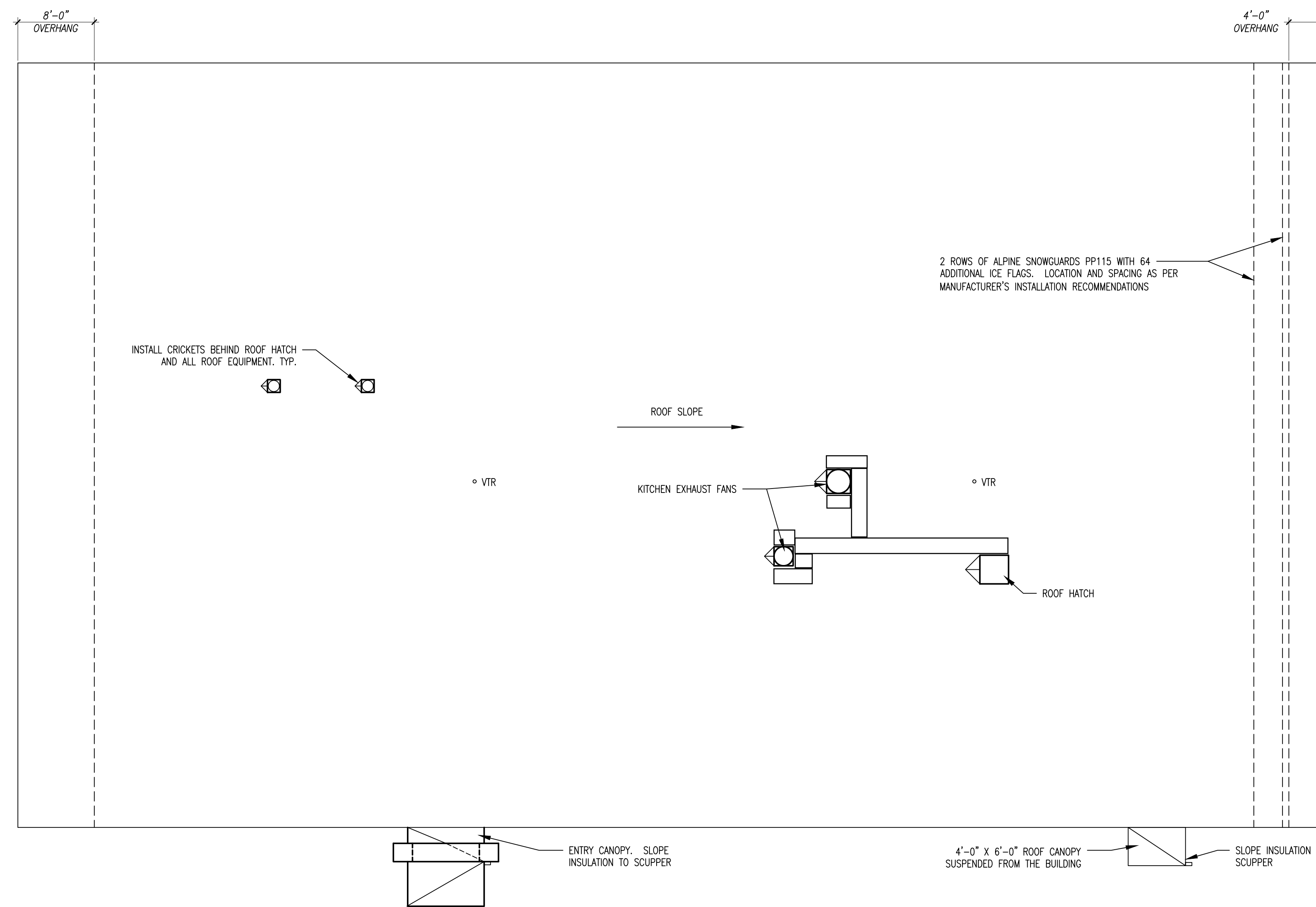
01 ROOF PLAN SCALE: 1/8" = 1'-0"
