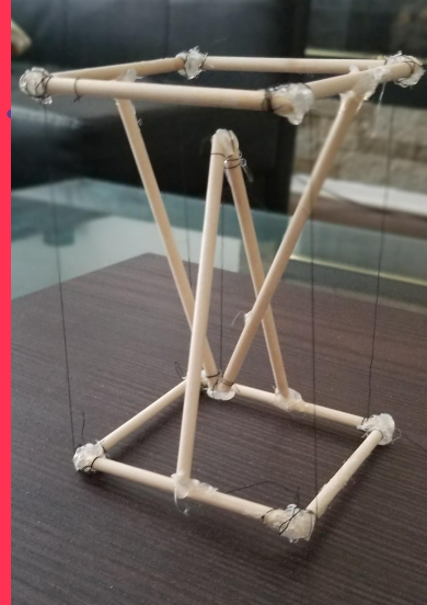
Tensegrity Table
