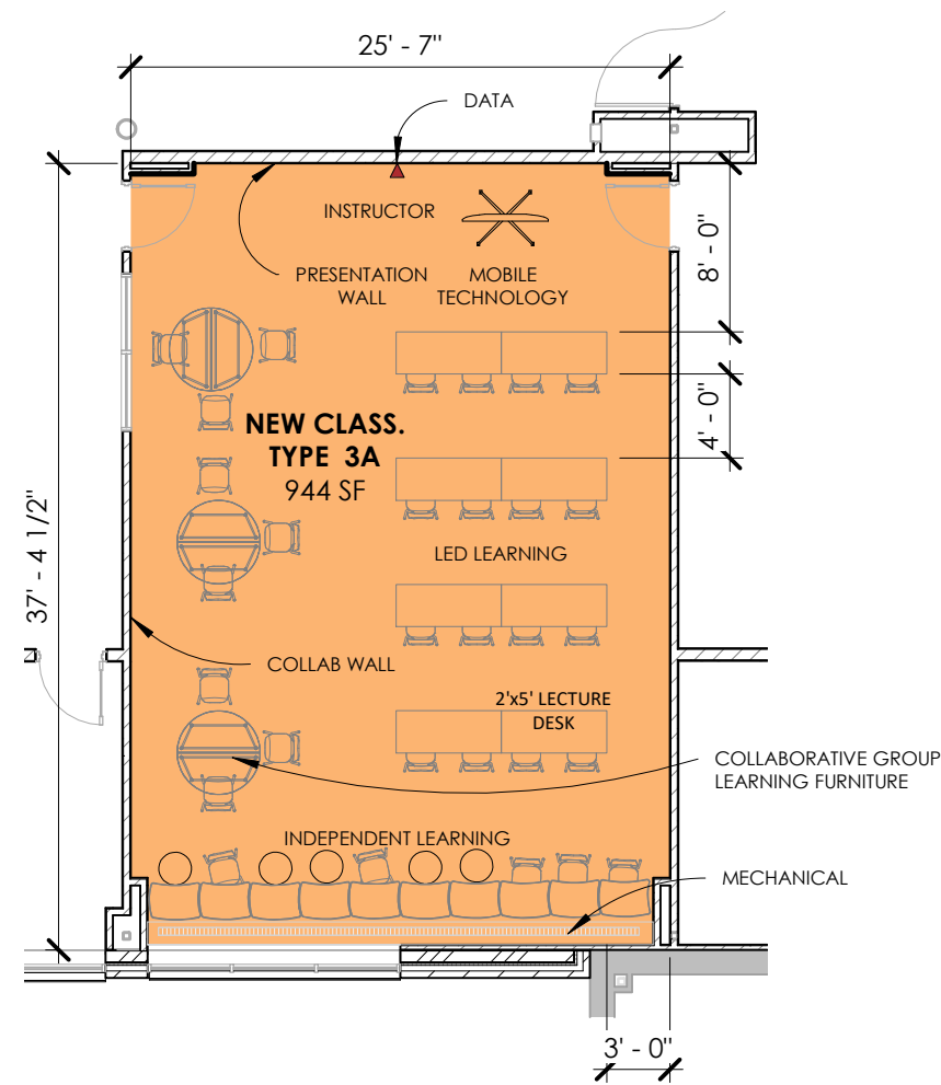
1- TYPE 3A
