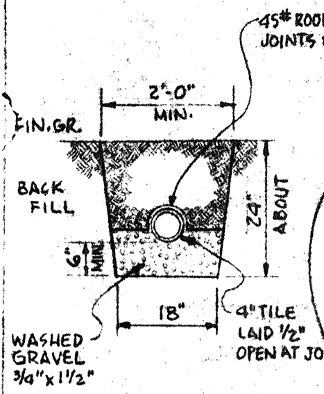
SECTION THRU DRAIN TRENCH SCALE: 1/2" = 1'-0"
